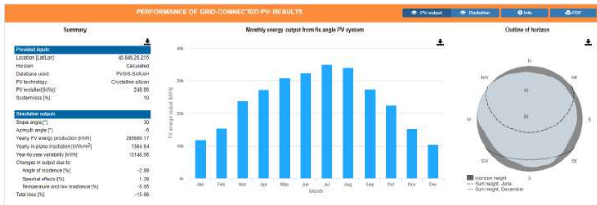
Fig. 3.4 – Simularea sistemului PV monocristalin – module 450 Wp + invertor 100 kWp pentru CEF TTS Covasna
